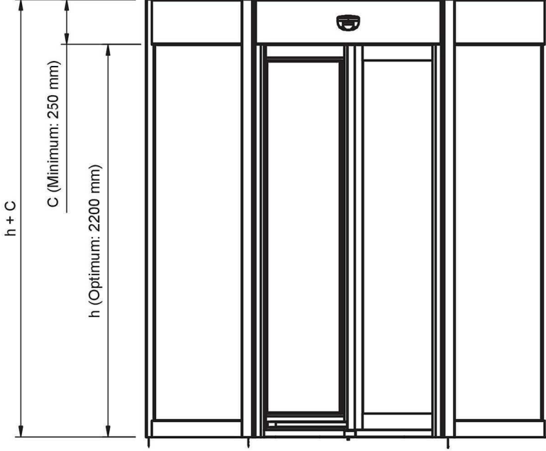
3 Kanatlı Otomatik Döner Kapı Standart Ölçüler 3 Wings Automatic Revolving Door Standard Dimensions
